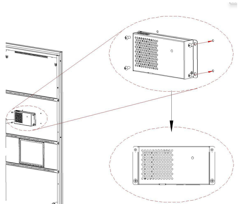
Рисунок 5-15 Монтаж RCD
