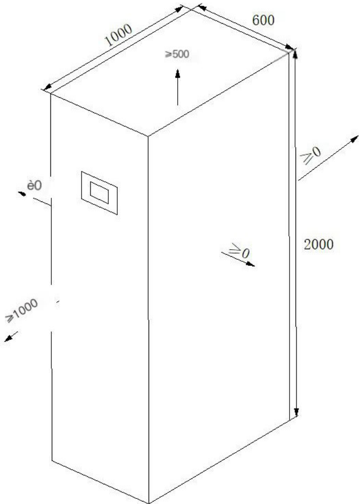
Рисунок 5-1 Схема пространства вокруг шкафа
