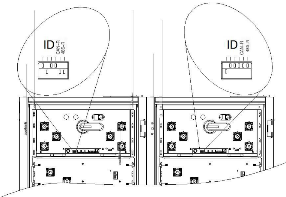
Рисунок 5-24 Многопозиционный переключатель
