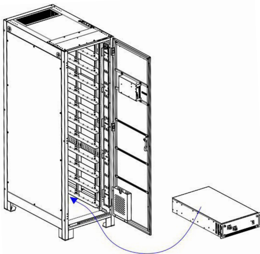
Рисунок 5-10 Монтаж модуля / CBMS в шкаф
